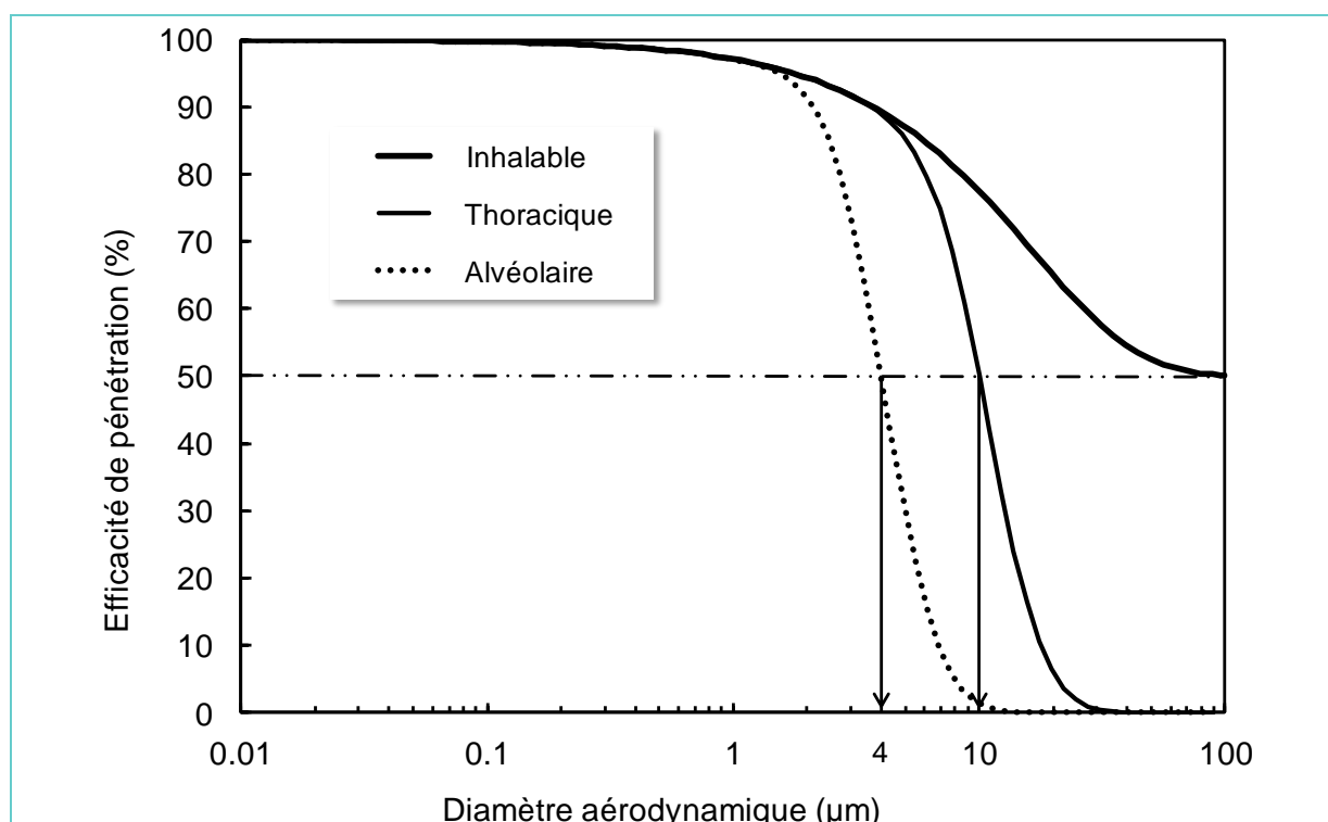
Figure 1 : Courbes conventionnelles CEN [1] définissant les fractions inhalable, thoracique et alvéolaire d'un aérosol en fonction du diamètre équivalent aérodynamique des particules.
